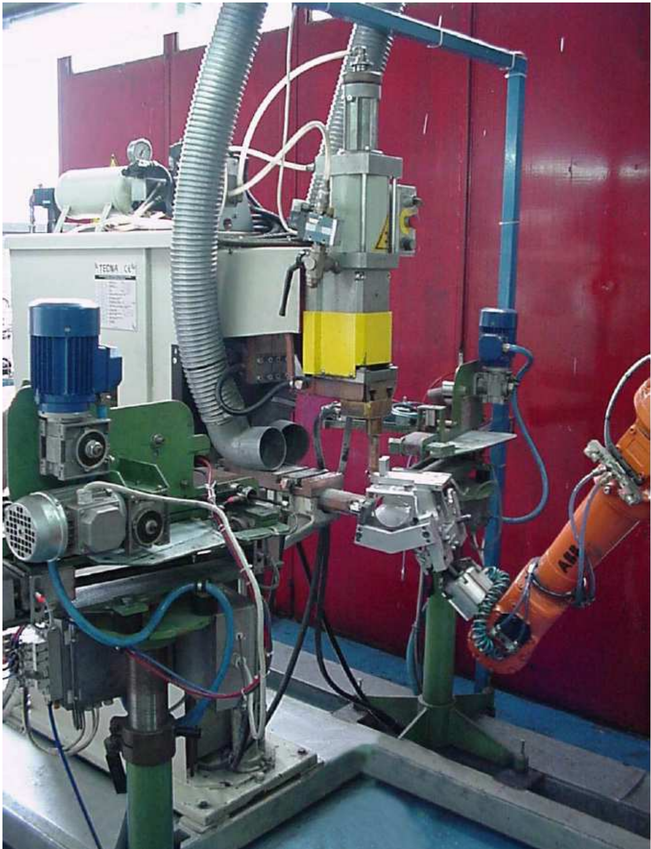
PUNKT APARAT U KOMBINACIJI SA ROBOTSKOM RUKOM
